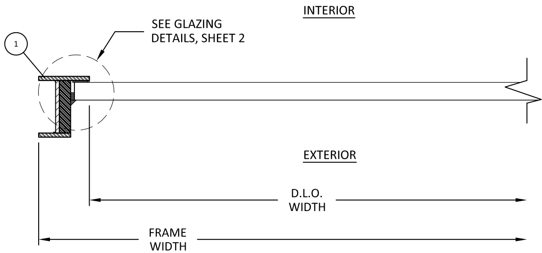
A 6 HORIZONTAL SECTION LEFT JAMB
