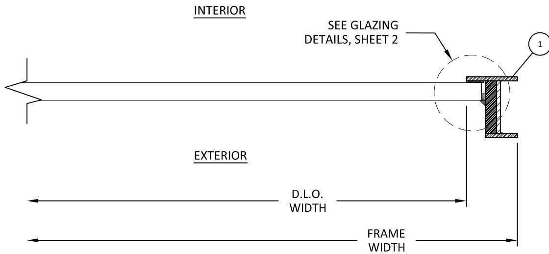
B 6 HORIZONTAL SECTION RIGHT JAMB
